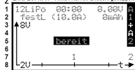
Z Bild 23.4.A1 Akku1 Kurven-Bildsch. gekoppelt
