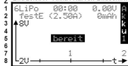
Z Bild 23.3.A1 Akku1 Kurven-Bildschirm
